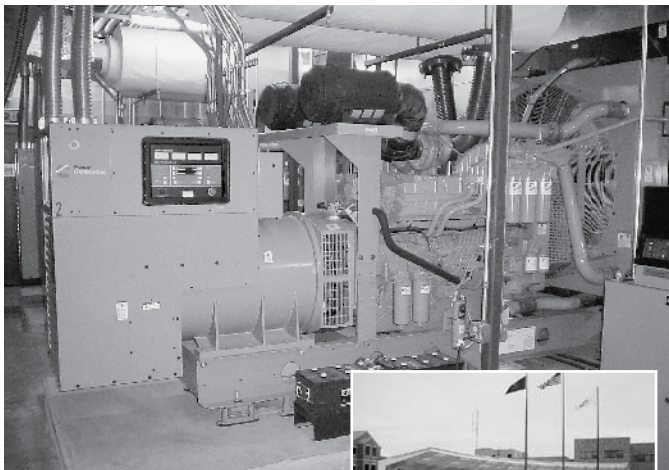
Dos grupos electrógenos de 1 MW proporcionan redundancia total a tres ramales energéticos en el Hancock Hospital, en Greenfield, Indiana.
